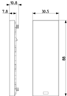
Vista ingombri
