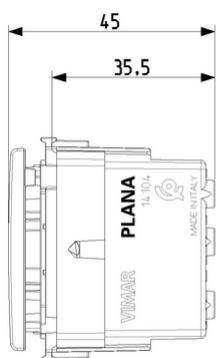
Vista ingombri
