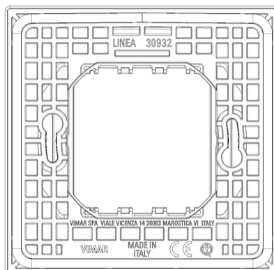
Vista posteriore
