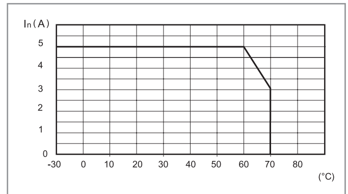
L78-17 Corrente di uscita in funzione della temperatura ambiente (78.W2)
