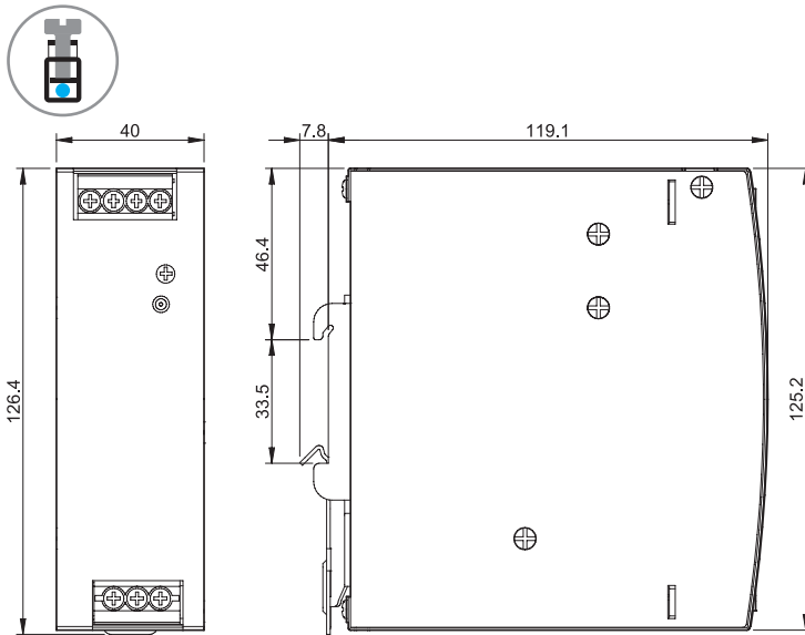
Tipo 78.X1 Morsetti a bussola
