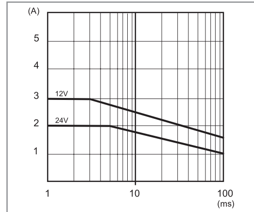
P78-2 Corrente di picco in funzione del tempo (78.12-xxxx)
