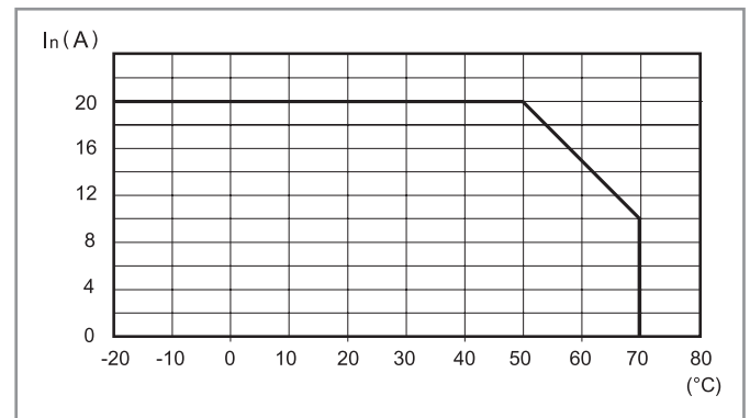
L78-15 Corrente di uscita in funzione della temperatura ambiente (78.Y1)
