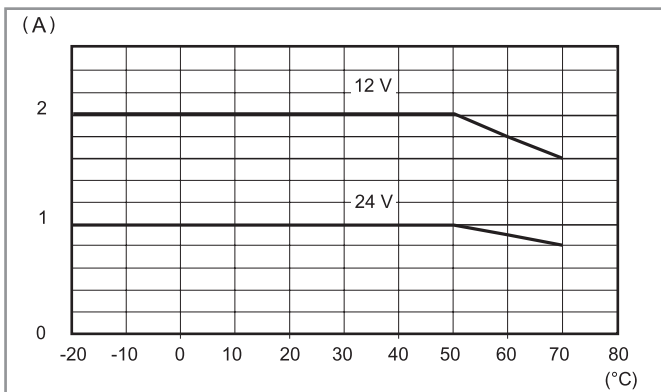
L78-3 Corrente di uscita in funzione della temperatura ambiente (78.25)
