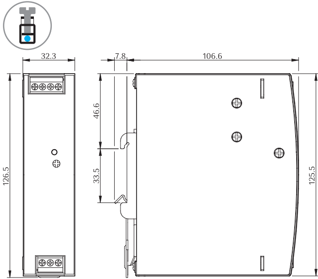
Tipo 78.W1 Morsetti a bussola
