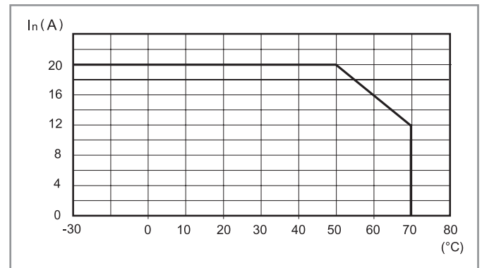
L78-19 Corrente di uscita in funzione della temperatura ambiente (78.Y2)
