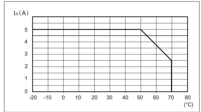
L78-13 Corrente di uscita in funzione della temperatura ambiente (78.W1)
