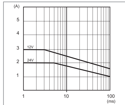
P78-3 Corrente di picco in funzione del tempo (78.25)
