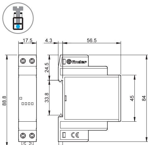
Tipo 78.12 Morsetti a bussola
