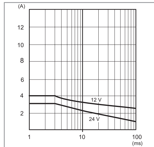
P78-3 Corrente di picco in funzione del tempo (78.25)
