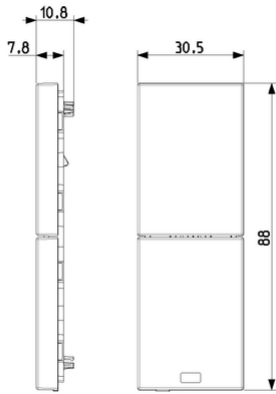
Vista ingombri
