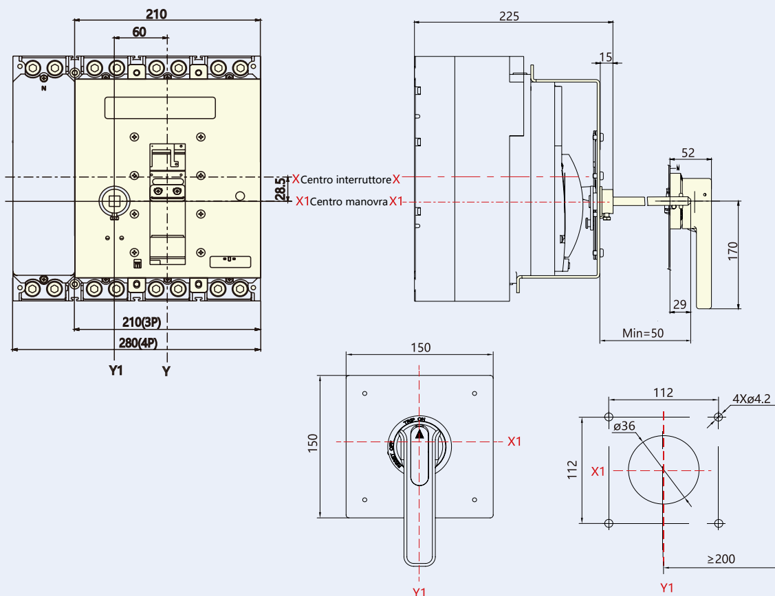
Dimensioni prodotto e di installazione SRH25-M8
