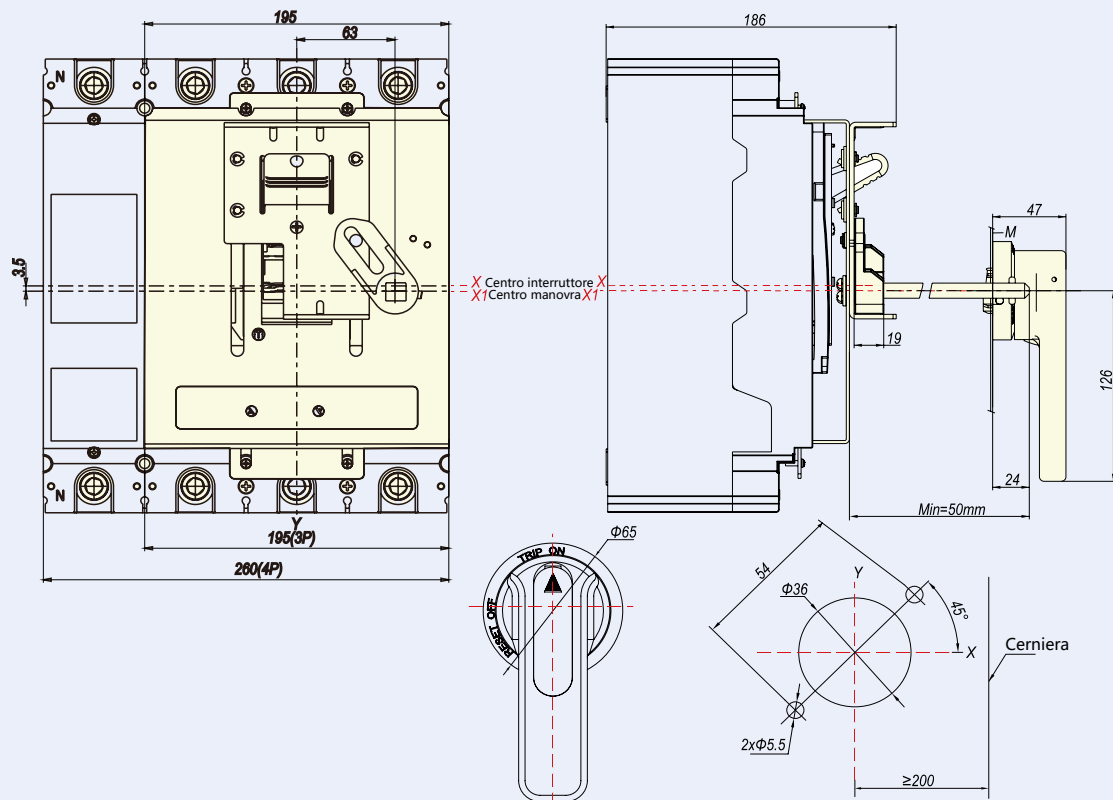
Dimensioni prodotto e di installazione SRH24-M8
