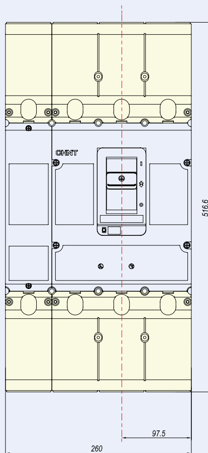
Copriterminale filo alto 4P
