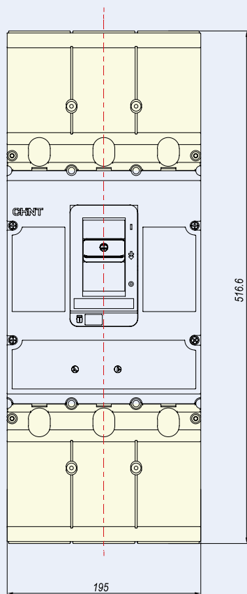
Copriterminale filo alto 3P
