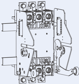
Installazione su guida DIN
